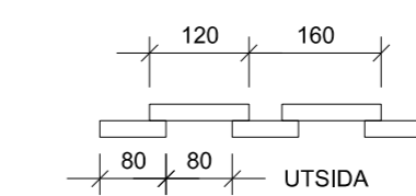
TYPDETALJ PANEL
