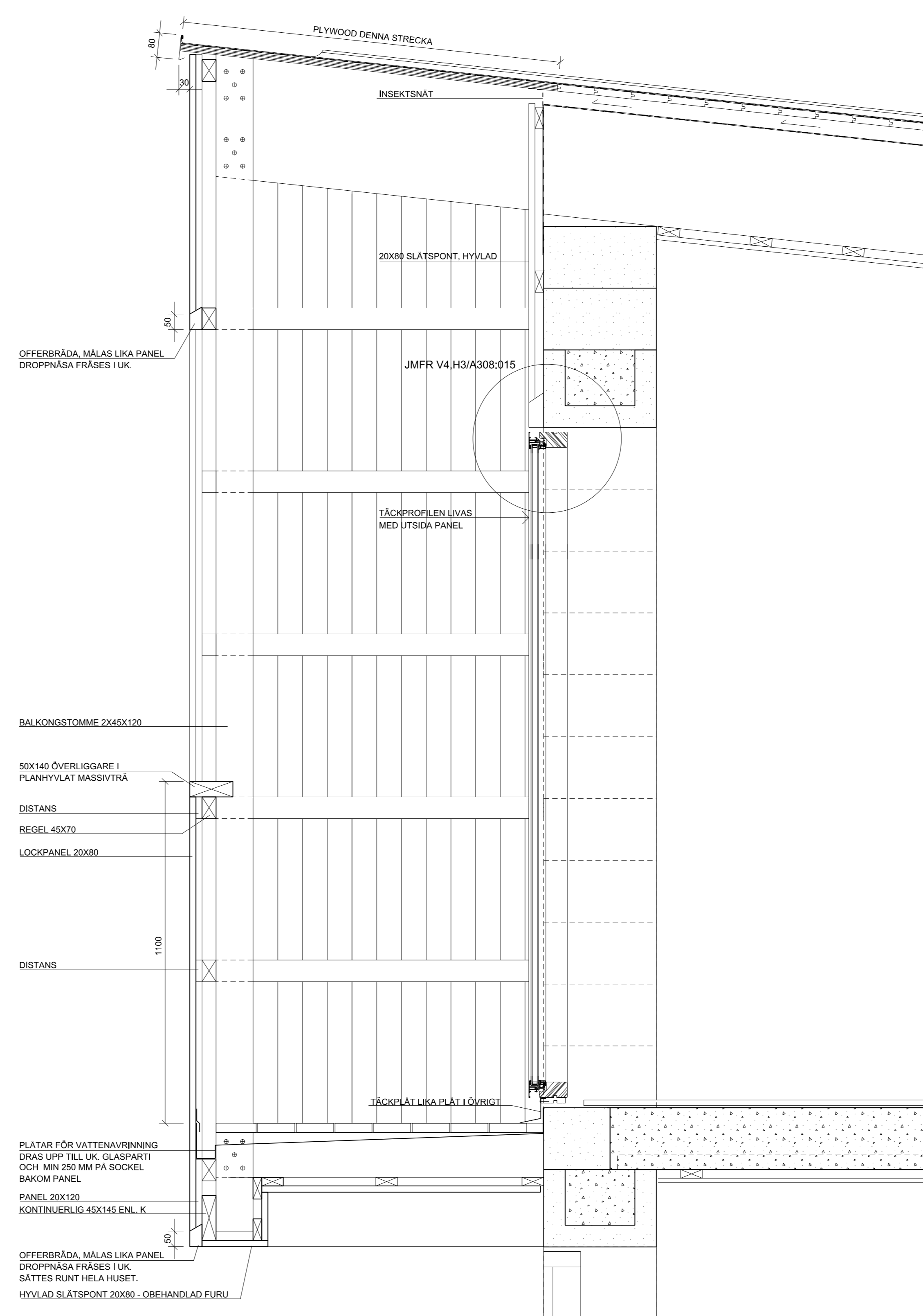
V1 SEKTION GENOM BALKONG
