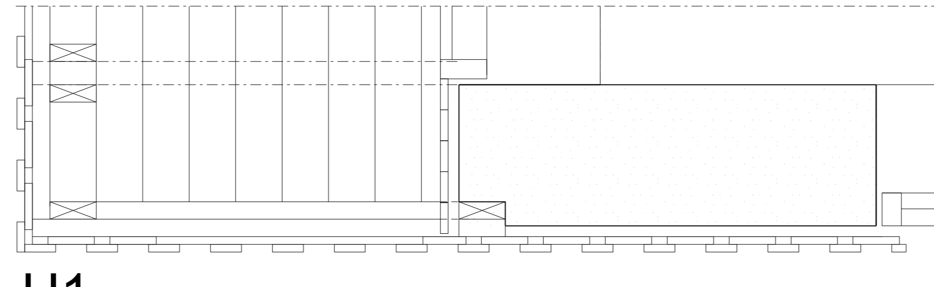
H1 SEKTION GENOM YTTERVÄGG/BALKONG
