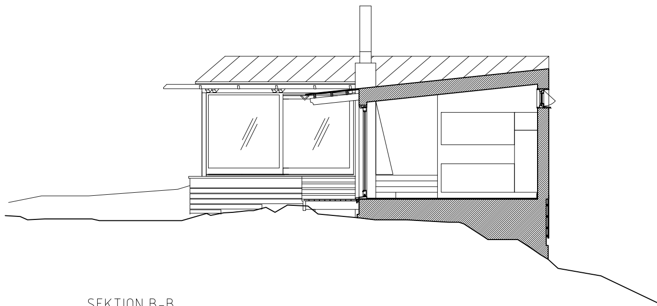
SEKTION B-B
