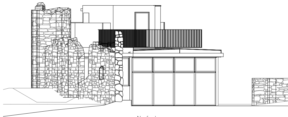
Norrfasad
