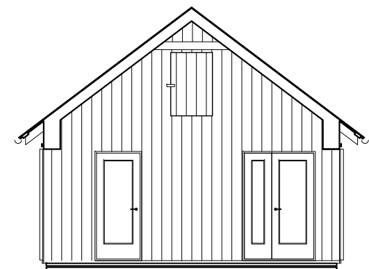
Sektion C-C
