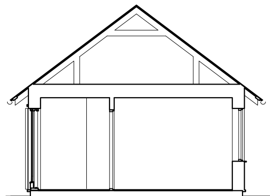
Sektion B-B
