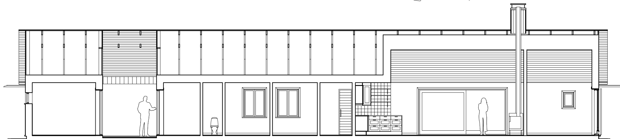
Sektion E-E
