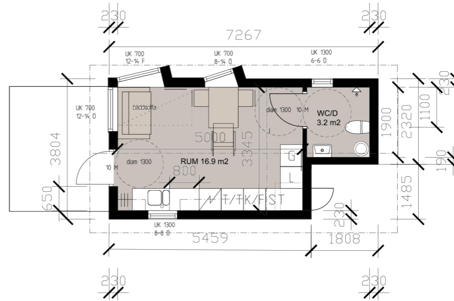
PLAN 1 1:100 A3, 1:50 A1
