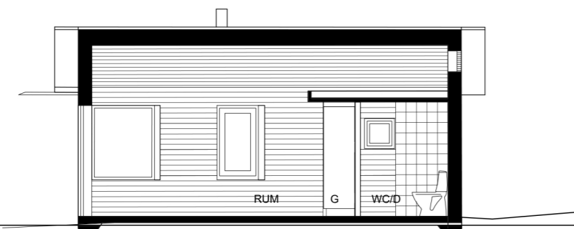
SEKTION B-B 1:100 A3, 1:50 A1
