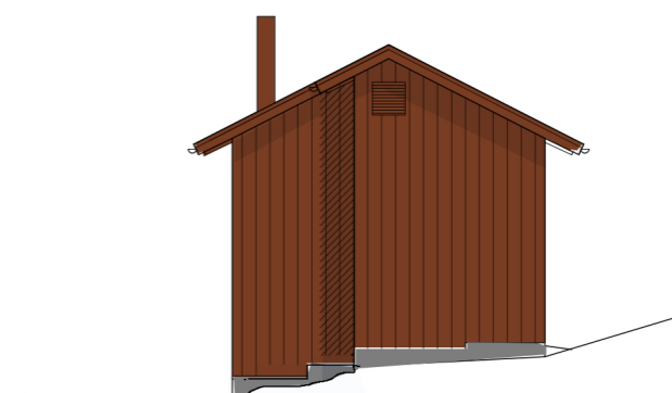
FASAD MOT NORR 1:100 A3, 1:50 A1
