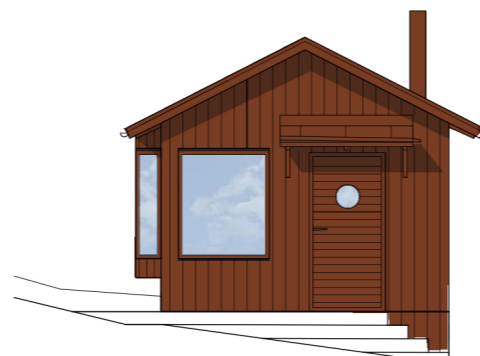
FASAD MOT SÖDER 1:100 A3, 1:50 A1
