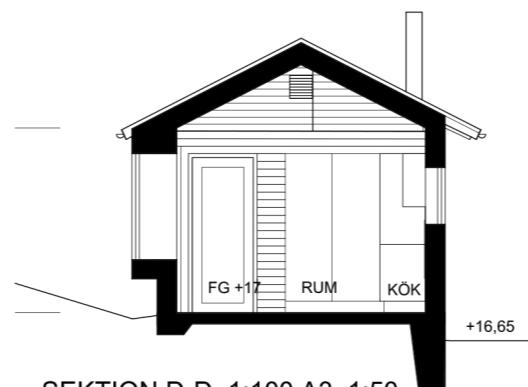
SEKTION D-D, 1:100 A3, 1:50 A1
