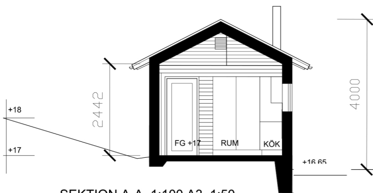
SEKTION A-A, 1:100 A3, 1:50 A1
