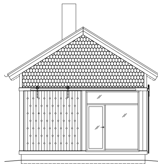
FASAD VÄST
