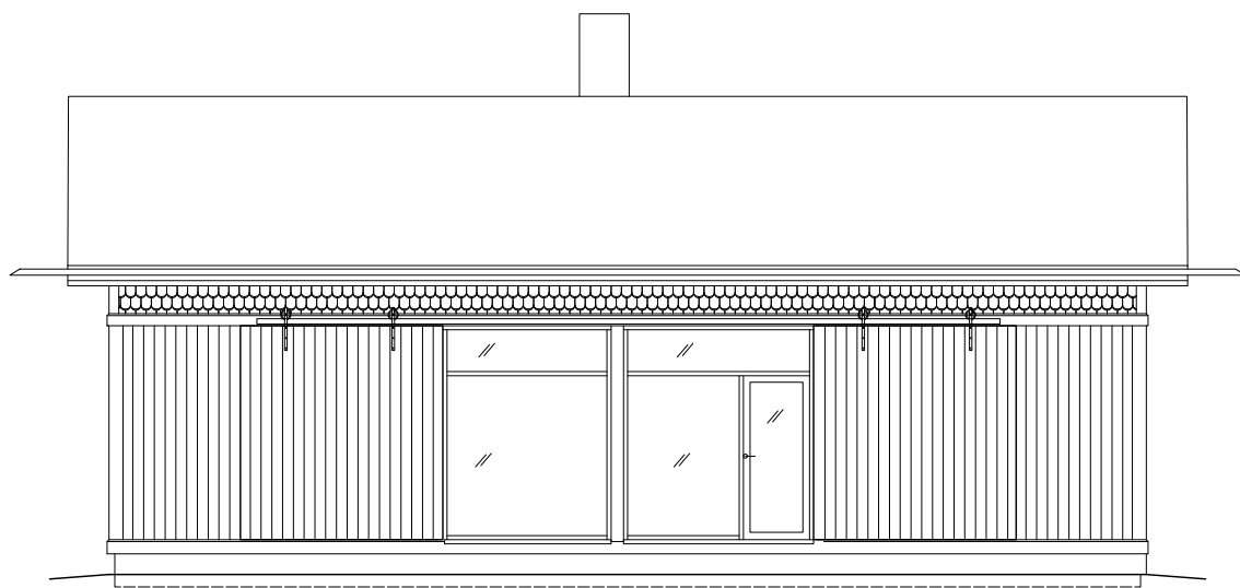
FASAD SYD
