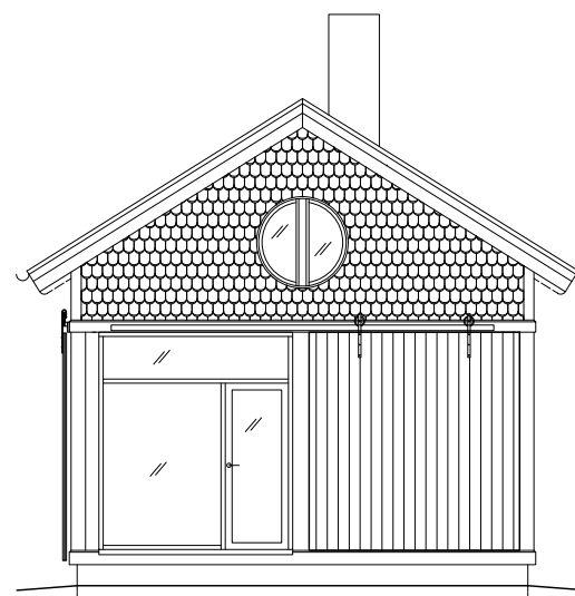
FASAD ÖST
