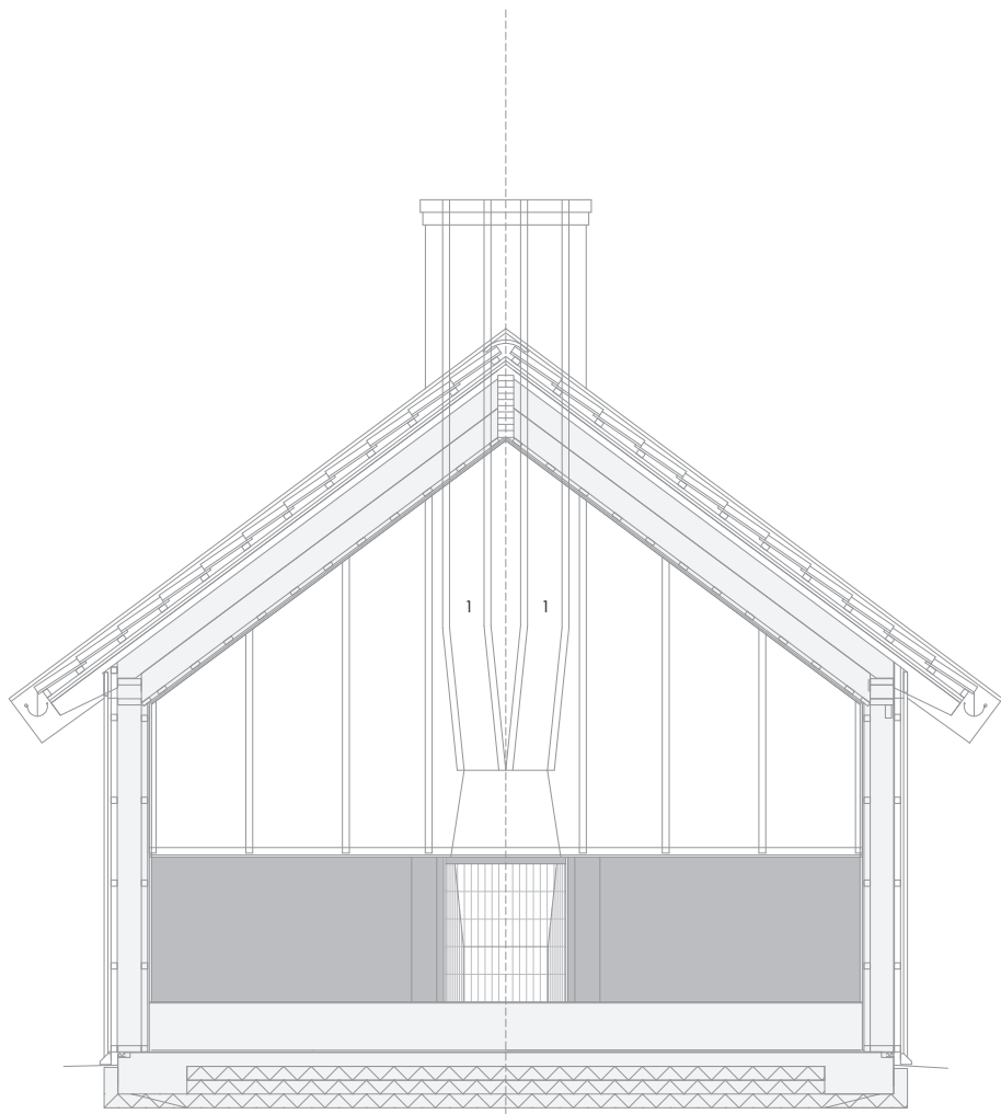
B-B
