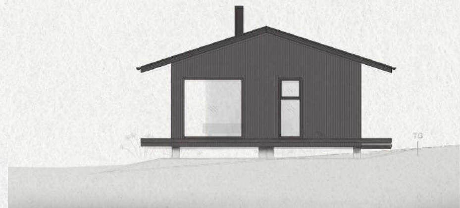
FASAD NORDÖST
