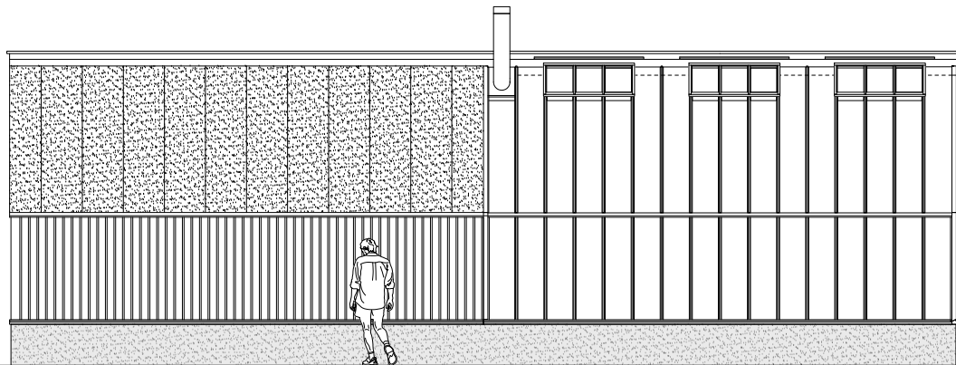
FASAD MOT SYD
