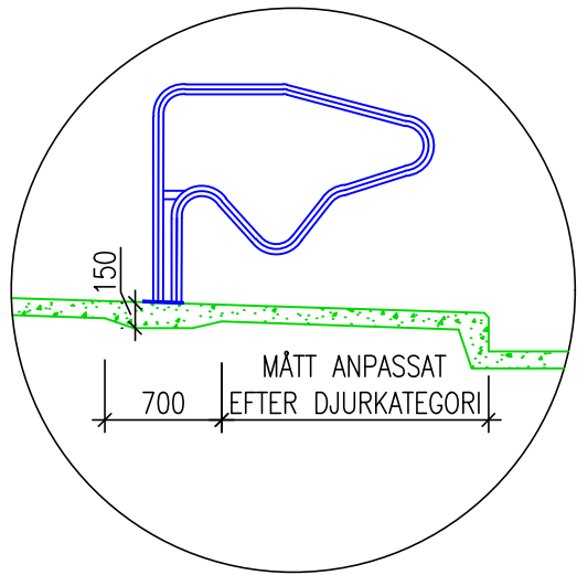
DETALJ A1 VOT UNDER LIGGBÅS SKALA 1:50
